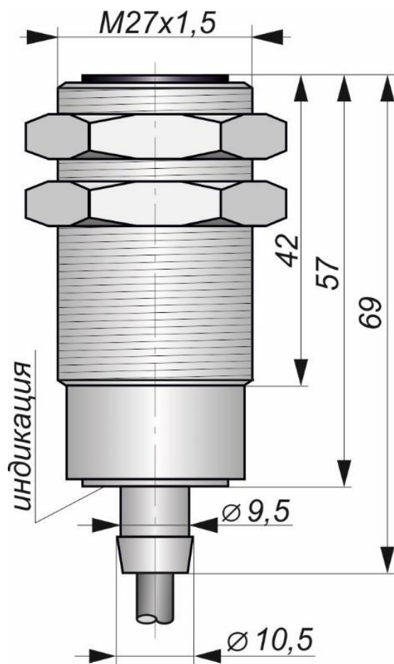
Габаритный чертеж
